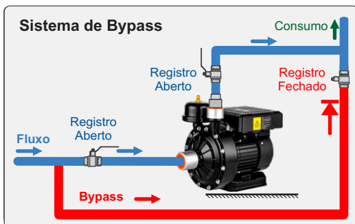
Figura 1 - Instalação em sistema de Bypass
